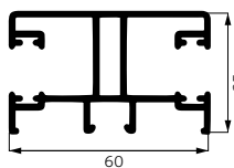
SR60A - Prowadnica aluminiowa dwukomorowa.
