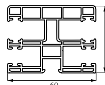
SRM60 - Prowadnica pvc dwukomorowa + moskitiera
