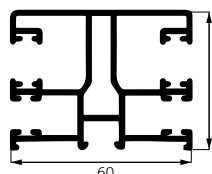
SRM60A - Prowadnica aluminiowa dwukomorowa + moskitiera
